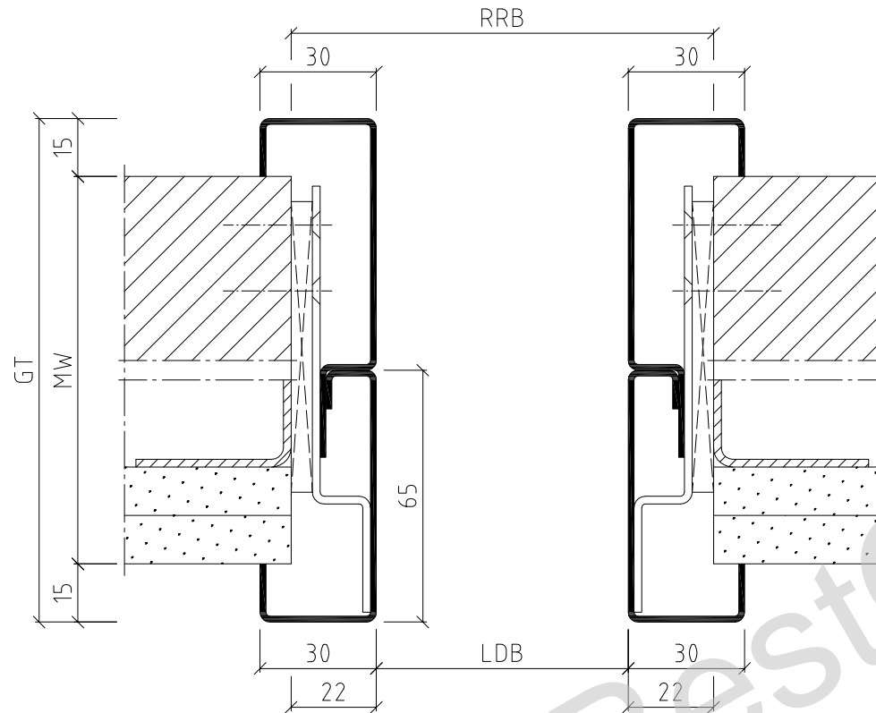
Horizontalschnitt
