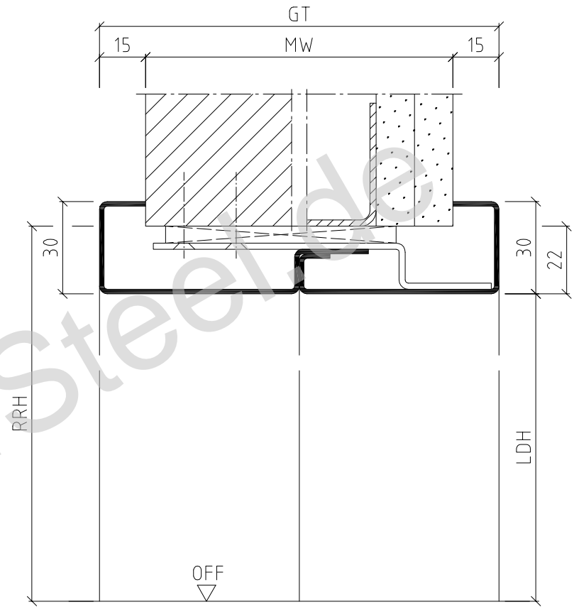
Vertikalschnitt
