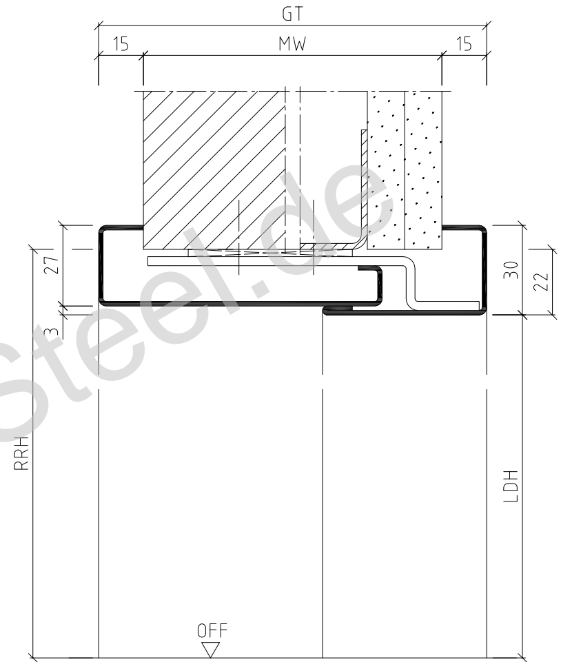
Vertikalschnitt
