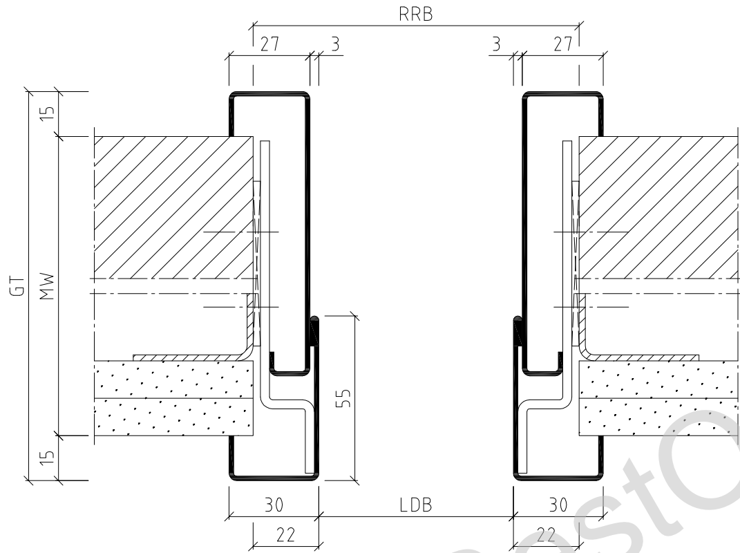
Horizontalschnitt
