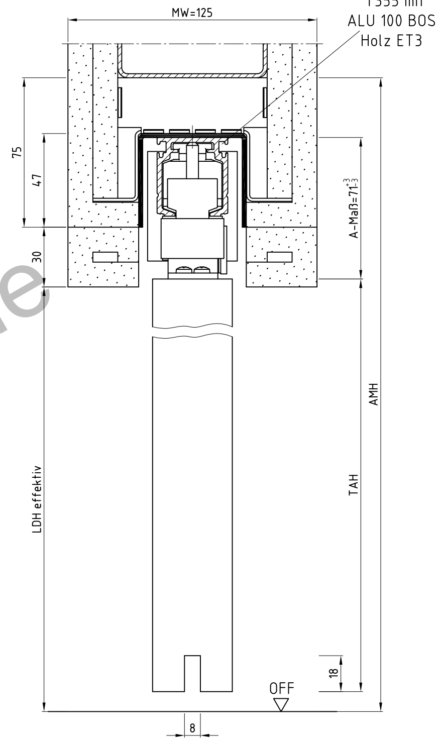
Schnitt B-B
