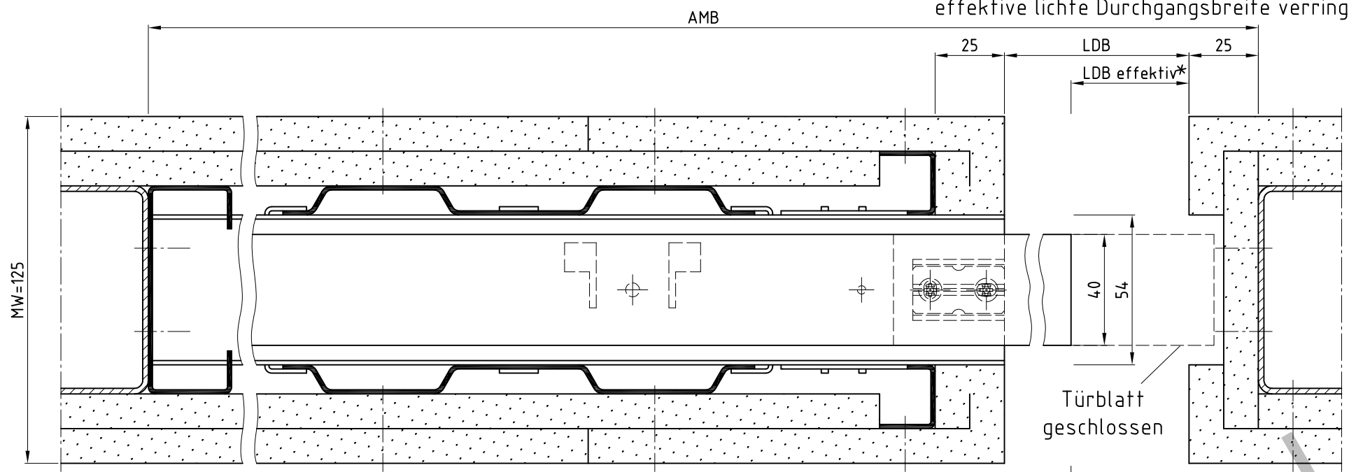
Schnitt A-A
