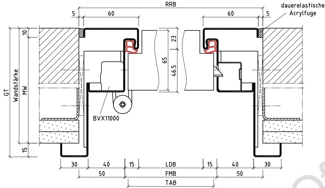
Horizontalschnitt
