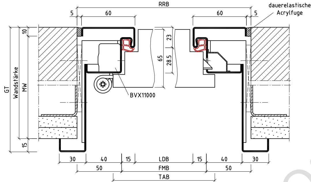
Horizontalschnitt
