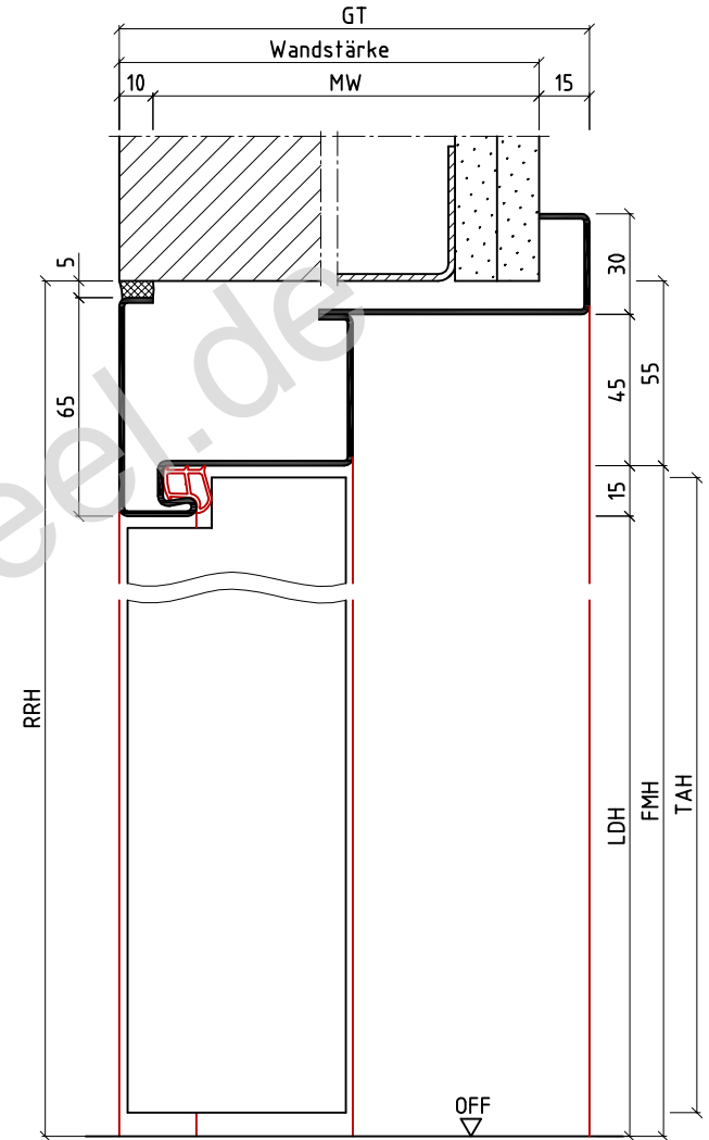
Vertikalschnitt
