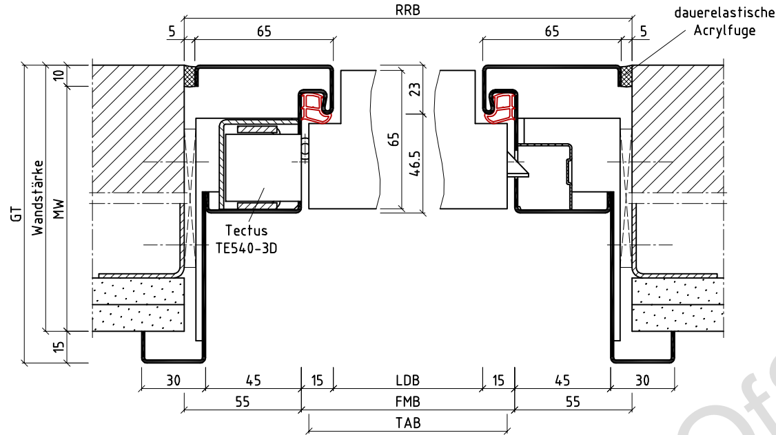
Horizontalschnitt
