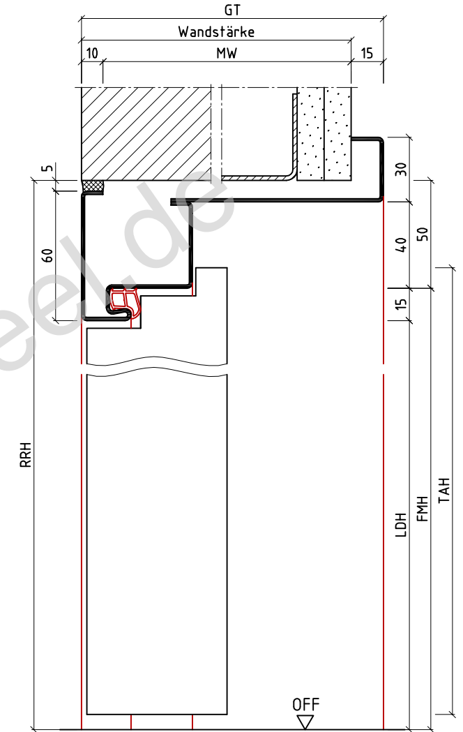
Vertikalschnitt
