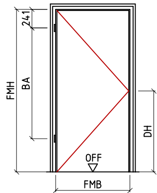
Ansicht: DIN links spiegelbildlich: DIN rechts
