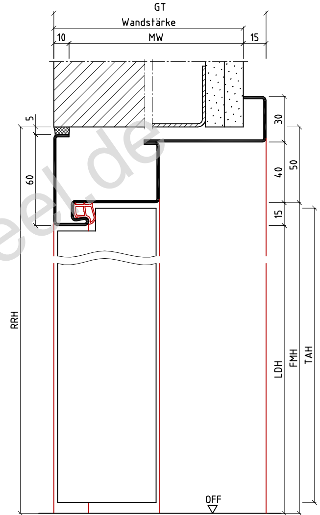
UA-Profil (gem. DIN 18182) bauseits, nach statischer Berechnung
