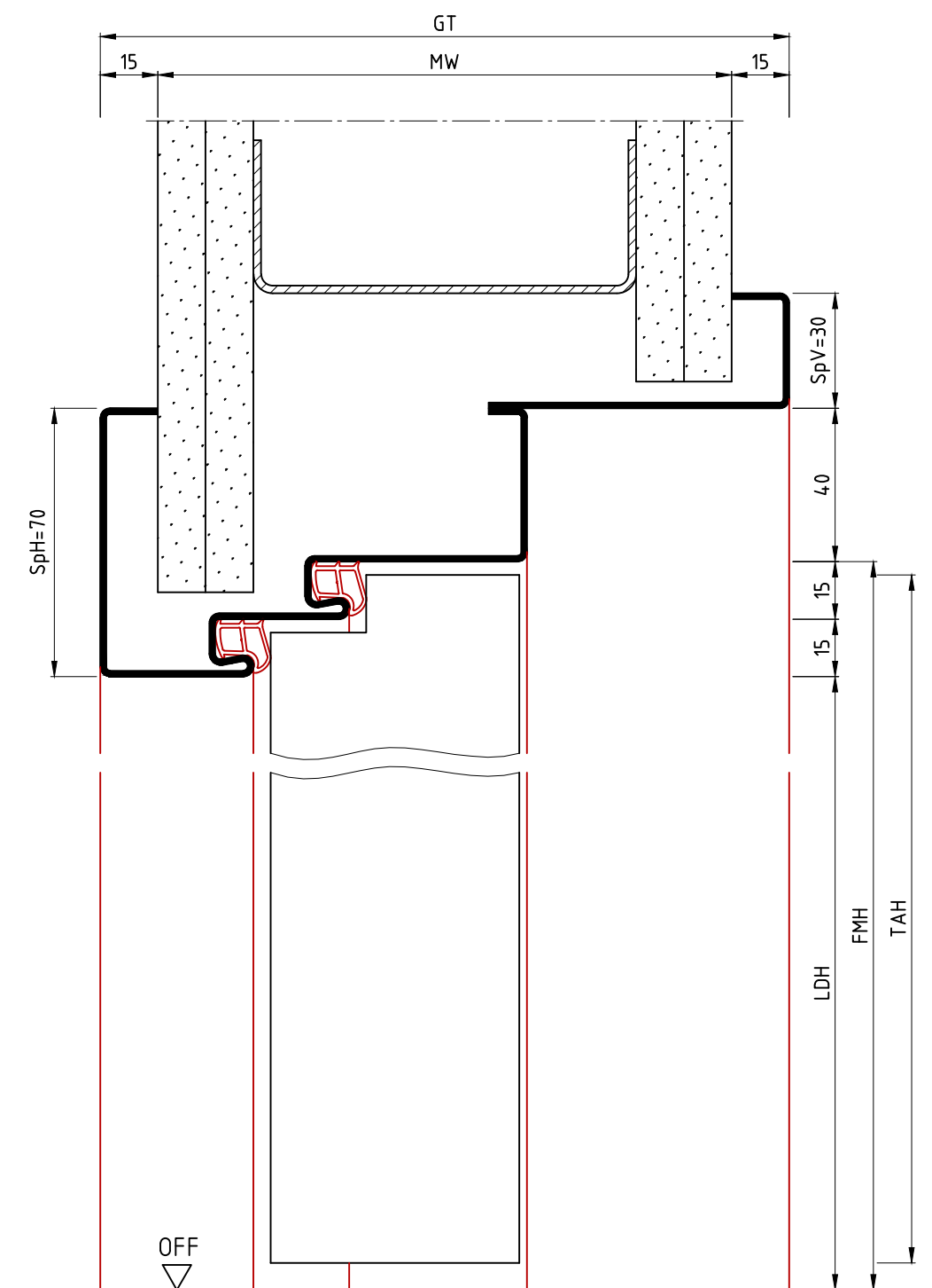
Vertikalschnitt
