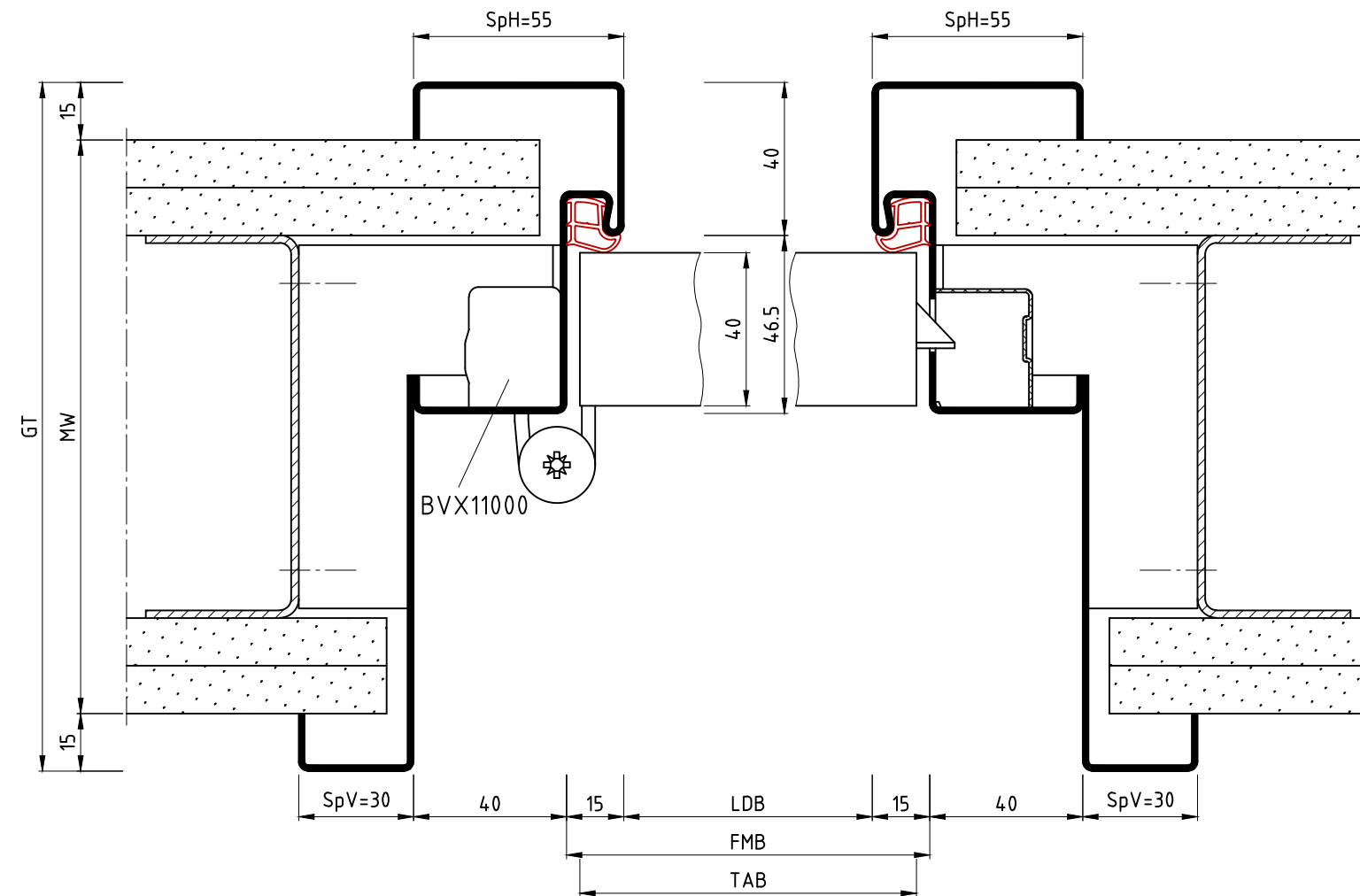
Horizontalschnitt
