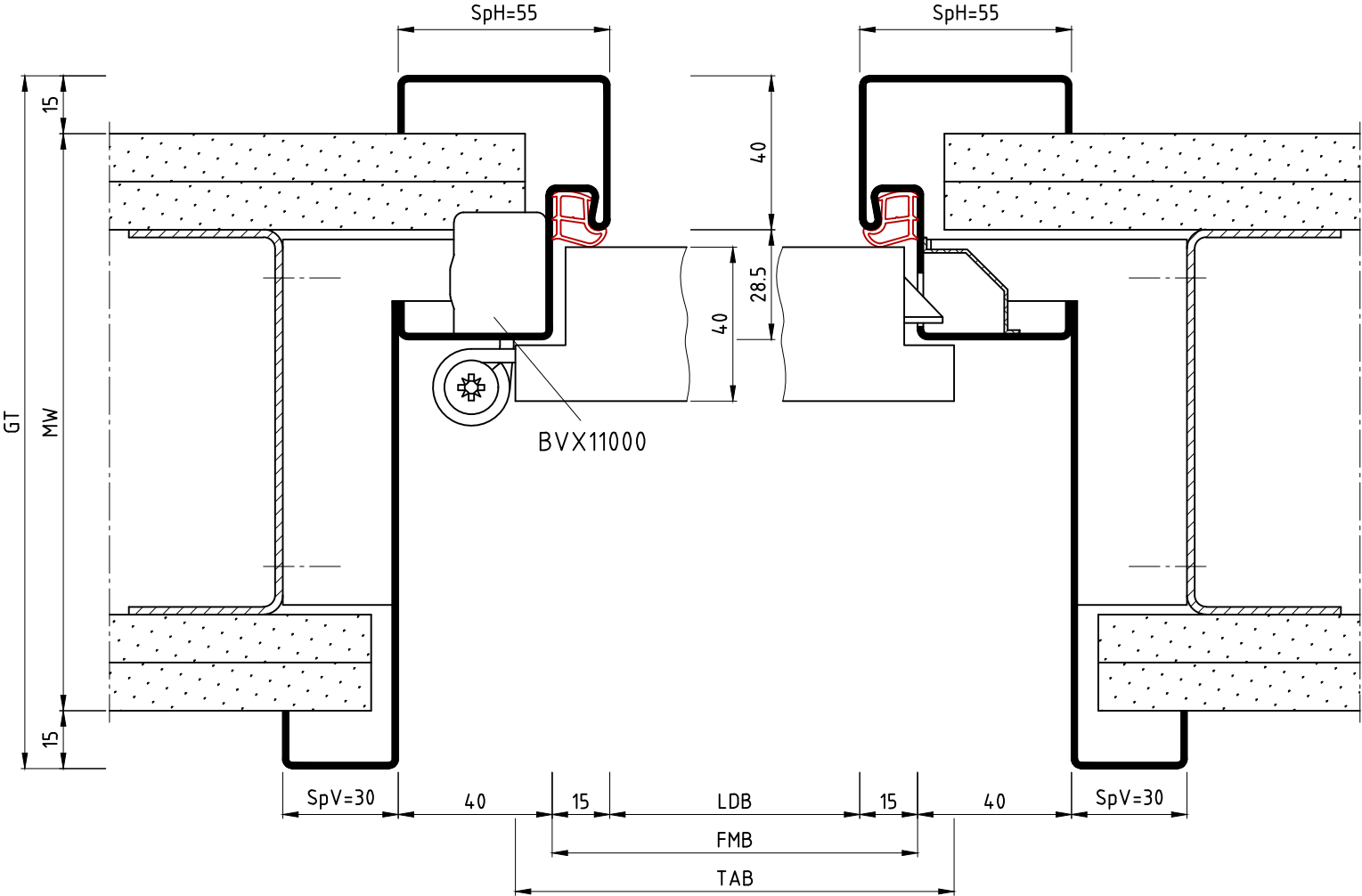
Horizontalschnitt
