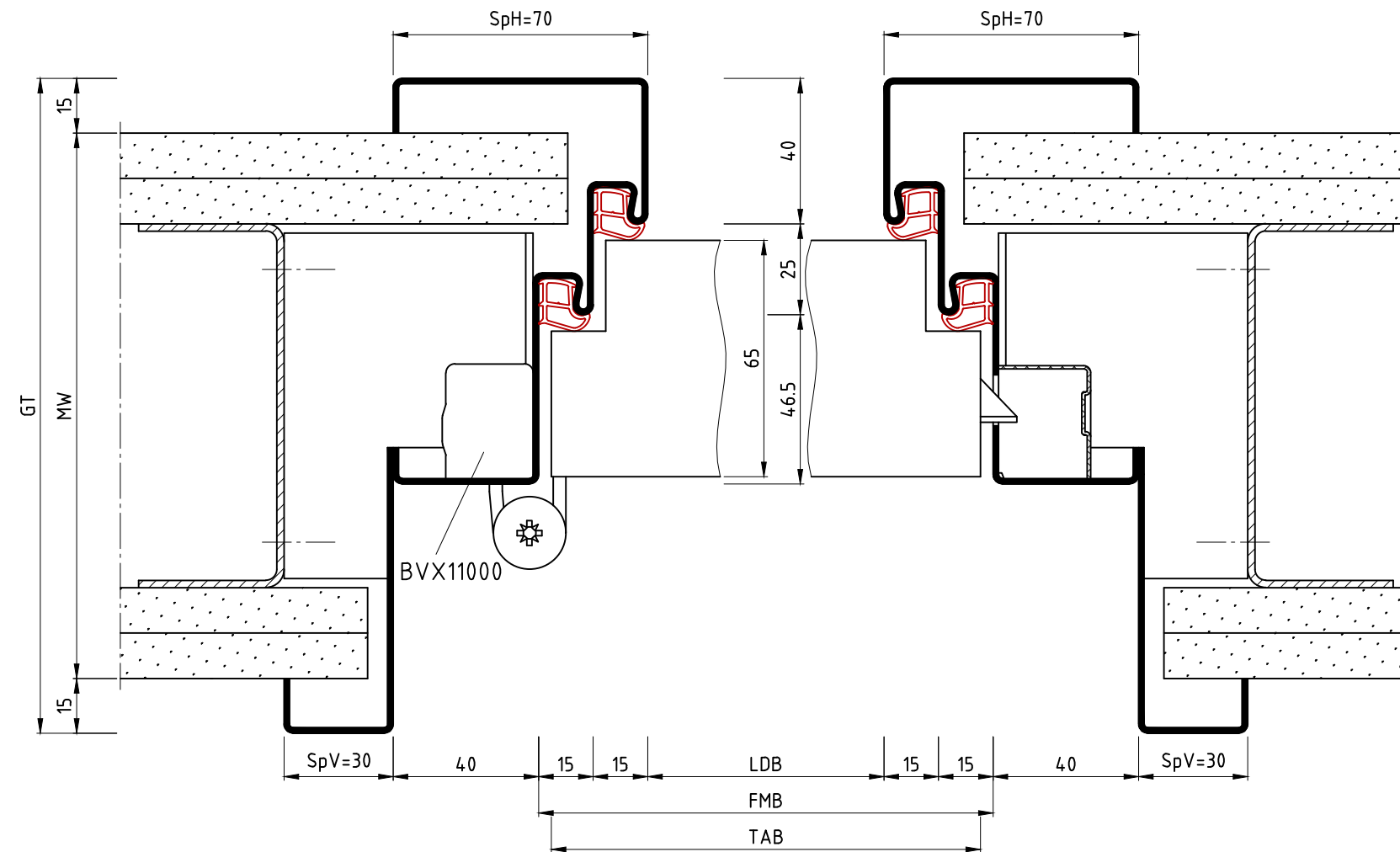
Horizontalschnitt
