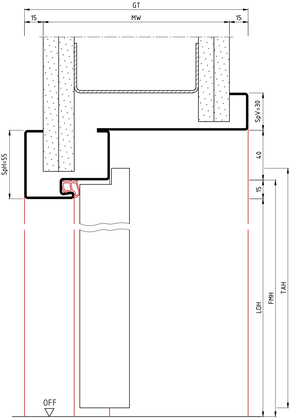
Vertikalschnitt
