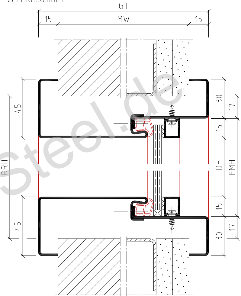
Vertikalschnitt
