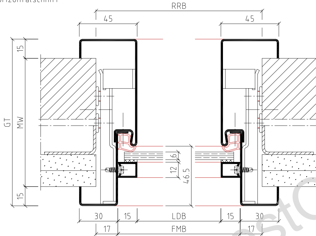
Horizontalschnitt
