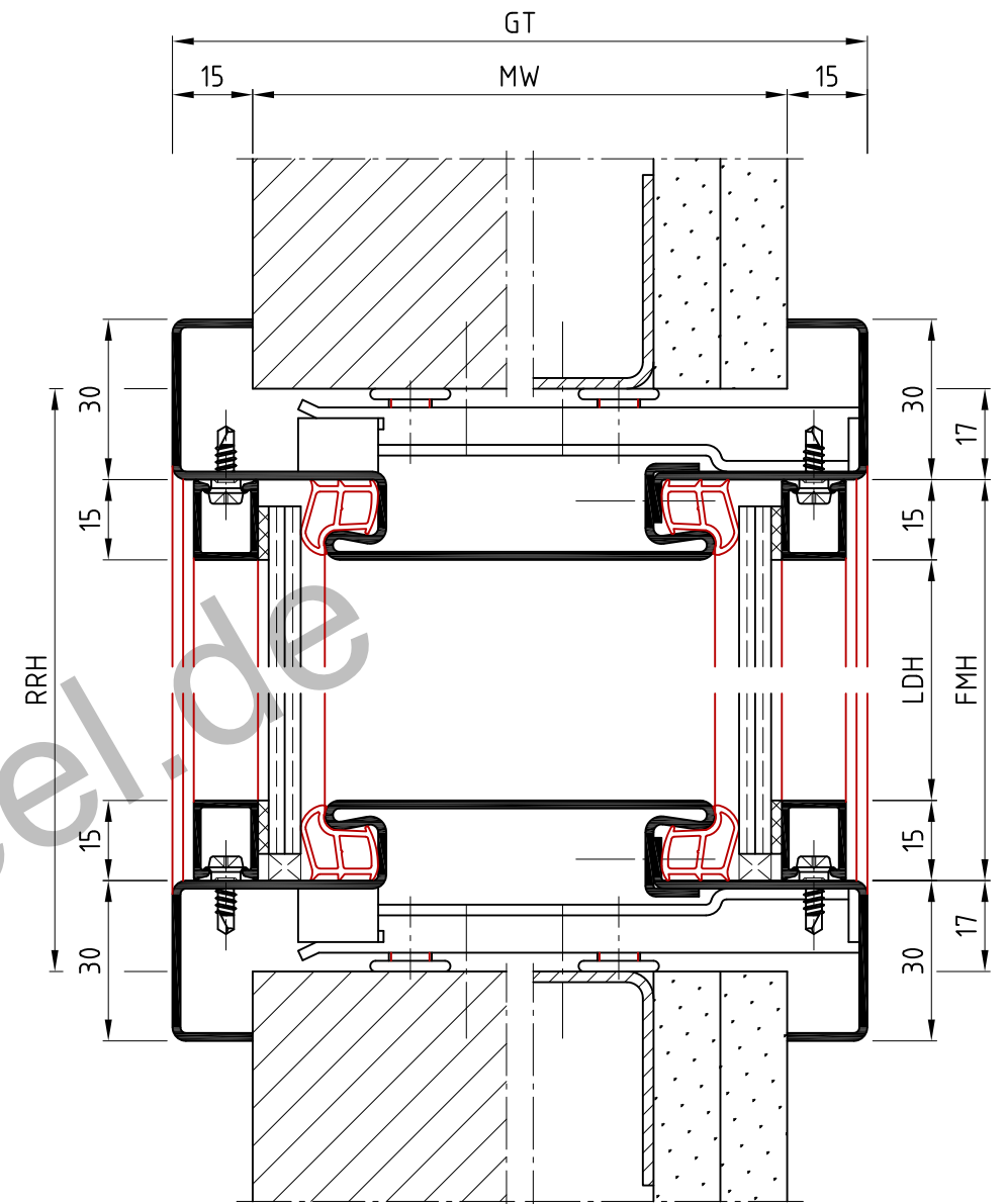
Schnitt B-B
