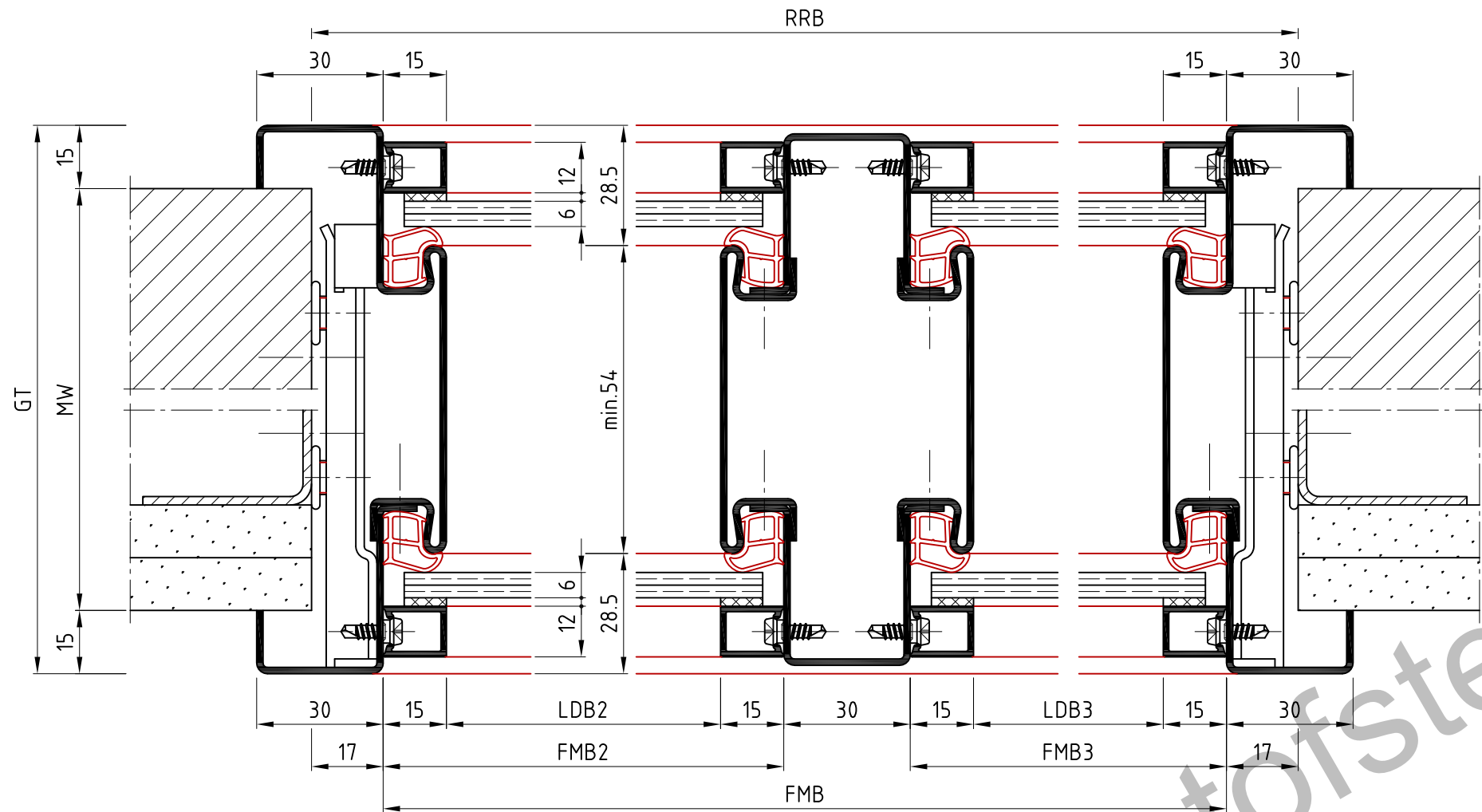
Schnitt A-A
