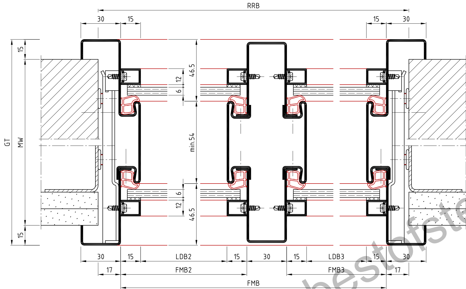
Schnitt A-A
