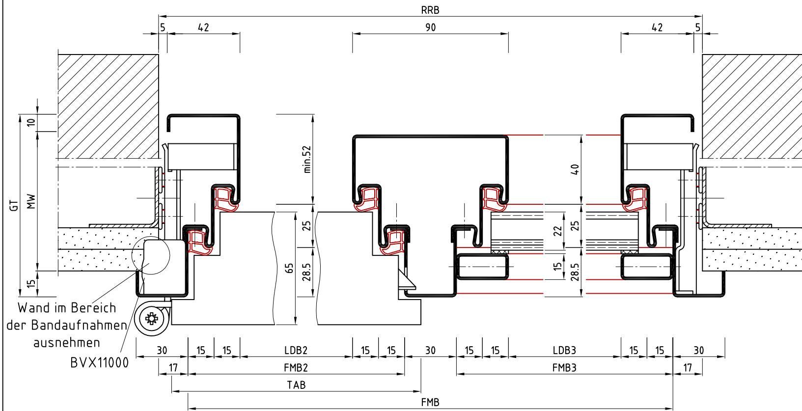
Schnitt A-A
