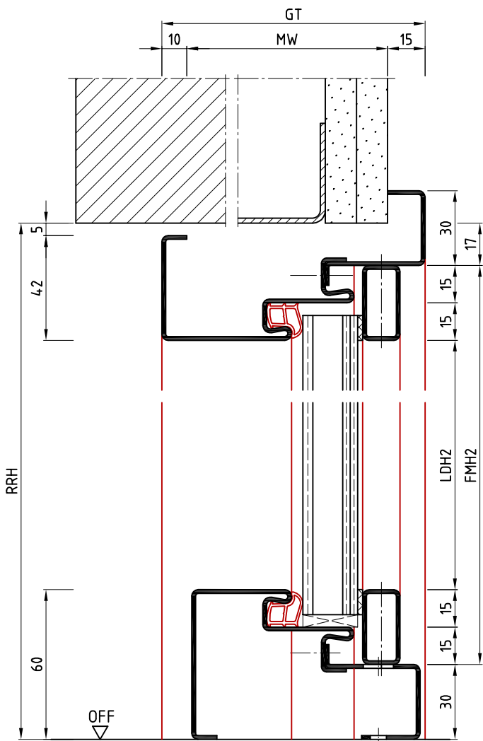
Schnitt C-C
