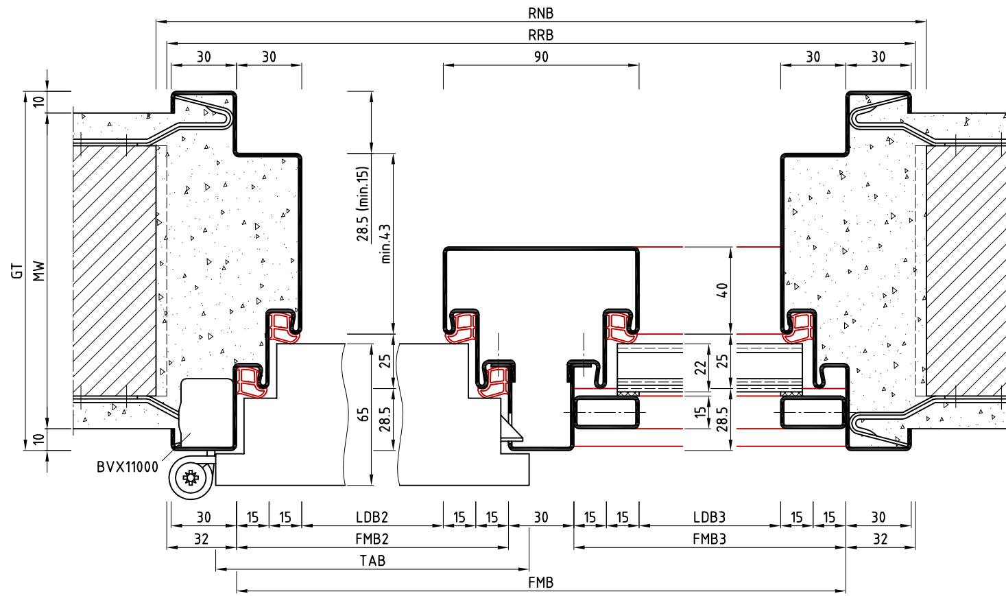
Schnitt A-A
