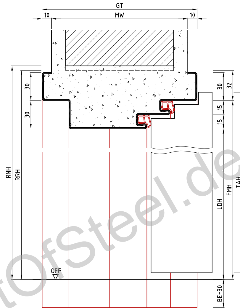
Schnitt B-B
