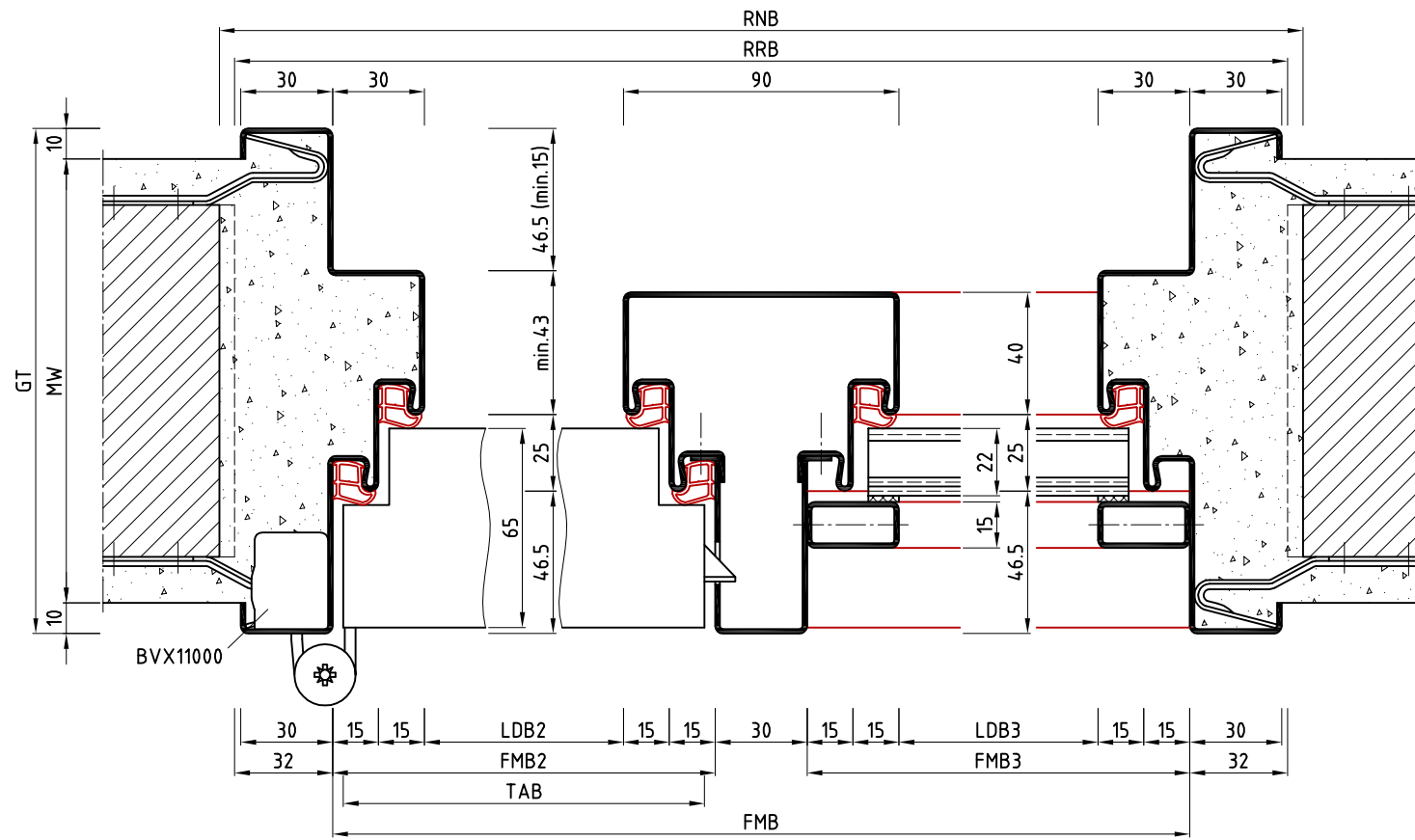
Schnitt A-A
