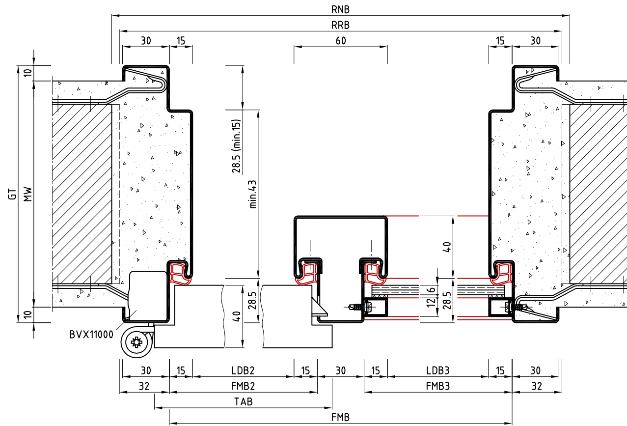
Schnitt A-A
