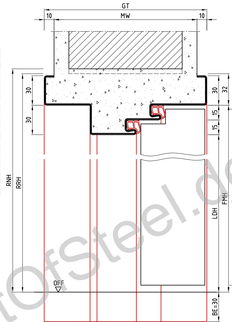
Schnitt B-B
