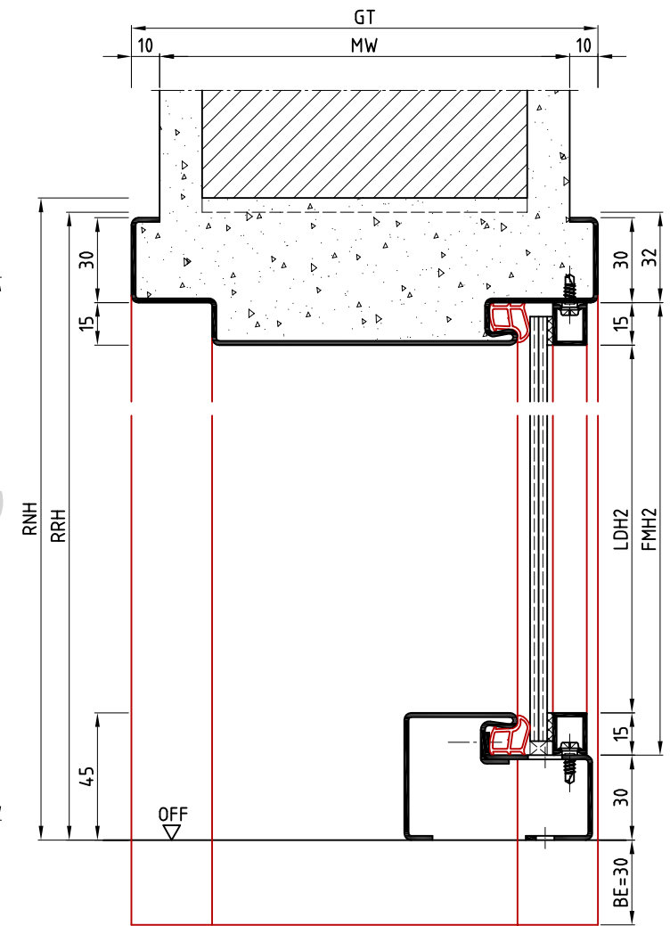
Schnitt C-C
