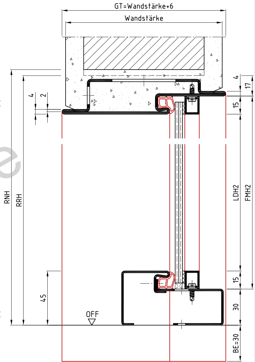
Schnitt C-C
