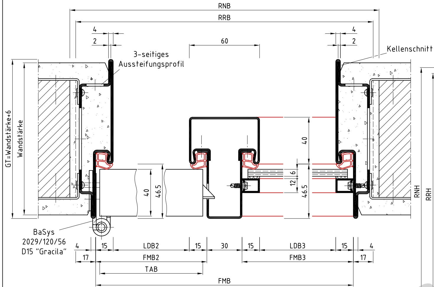
Schnitt A-A
