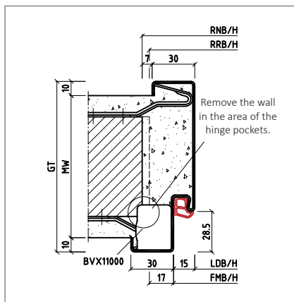
Non-standard frame similar to DIN 18111
