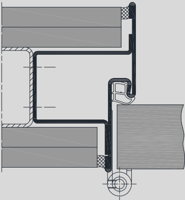
BaSys hinge
