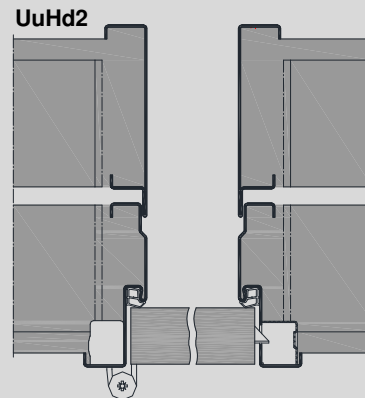
VX hinge
