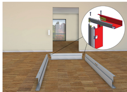
Dreiteilig und zerlegt: Die Stahlzarge Duo15Z ECON3 ab Lager. Bild 47c91344
