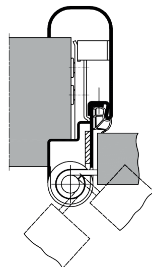
SafetyDesign: Der Türdrehpunkt ist mittig vom Spiegelradius. Bild 47c91342
