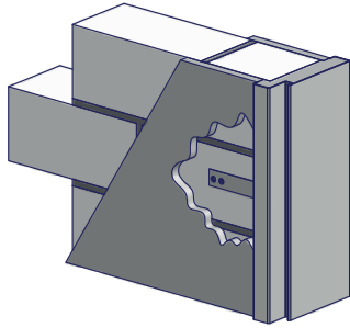
- Fester Nagel-/Dübelanker
