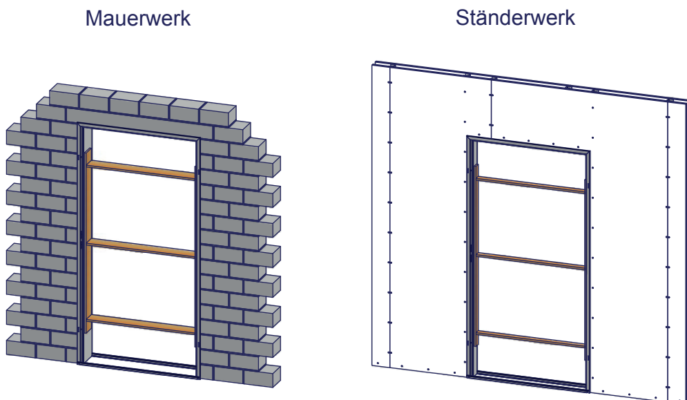
Bild 7 – Auffangen der Durchbiegung der Stahlzarge
