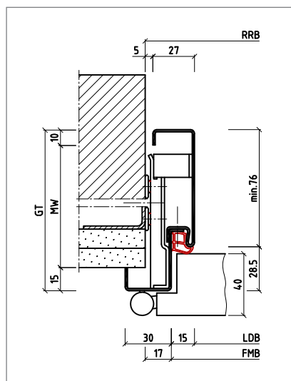
Eckzarge 15ZUud
