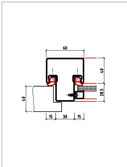
Eckkämpfer KEud
