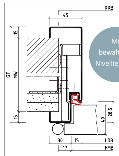
15ZBud
