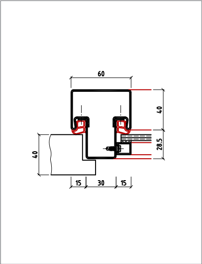
Eckkämpfer KEud
