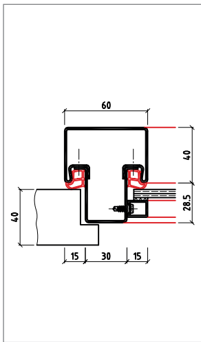
Eckkämpfer KEud
