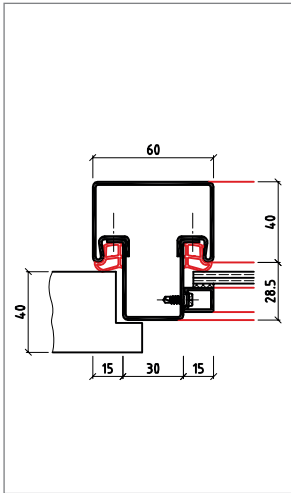
Eckkämpfer KEud
