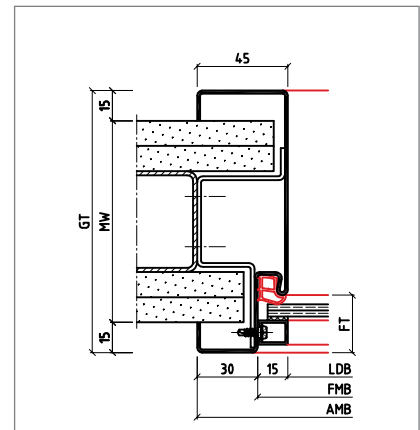
Bud (VGd)-Fensterzarge für Ständerwerk
