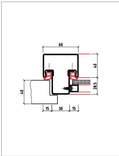
Eckkämpfer KEud
