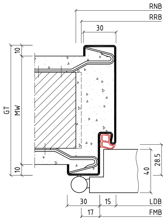
· Umfassungszarge (1-teilig) · für Mauerwerk · Darstellung mit Nagelanker
