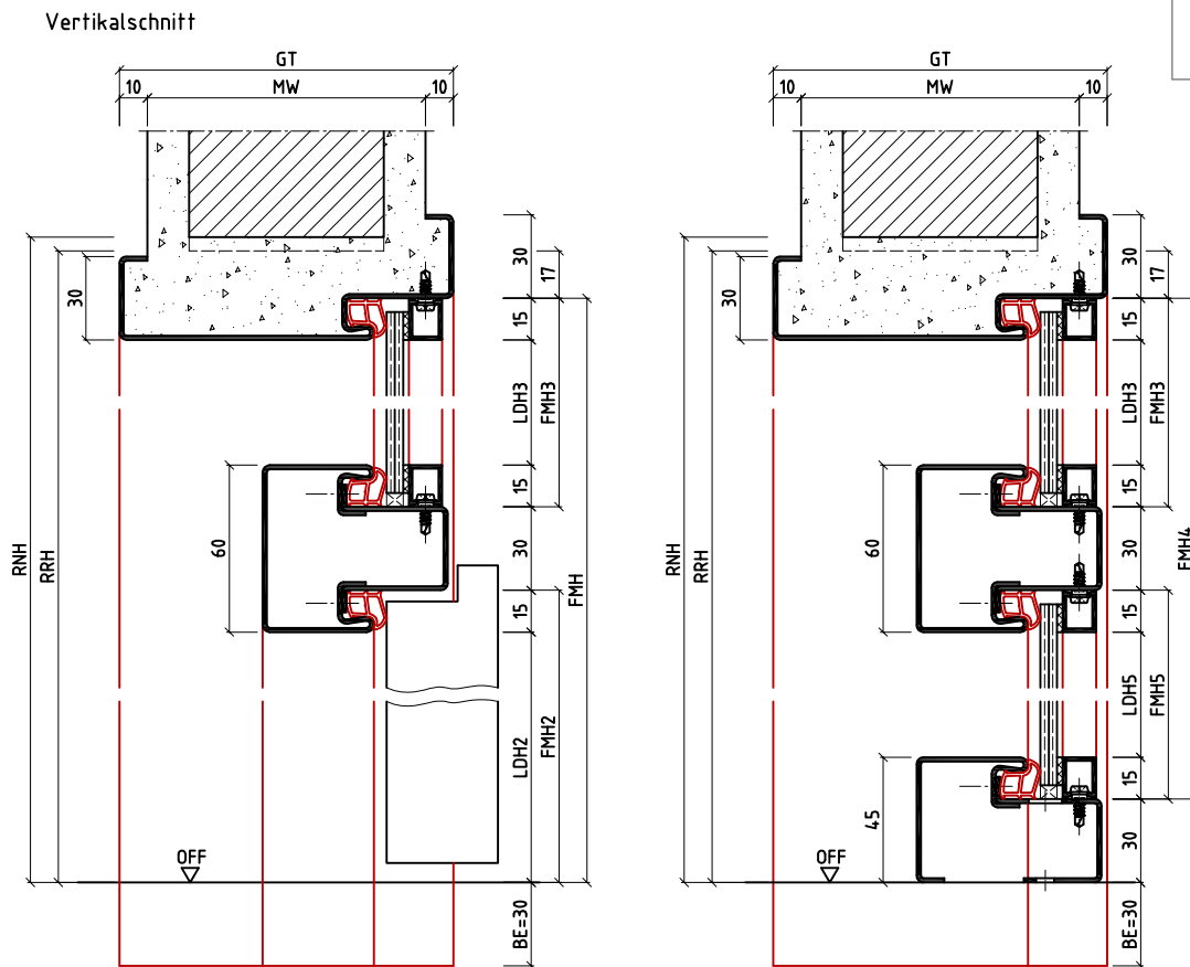
Darstellung Fall1
