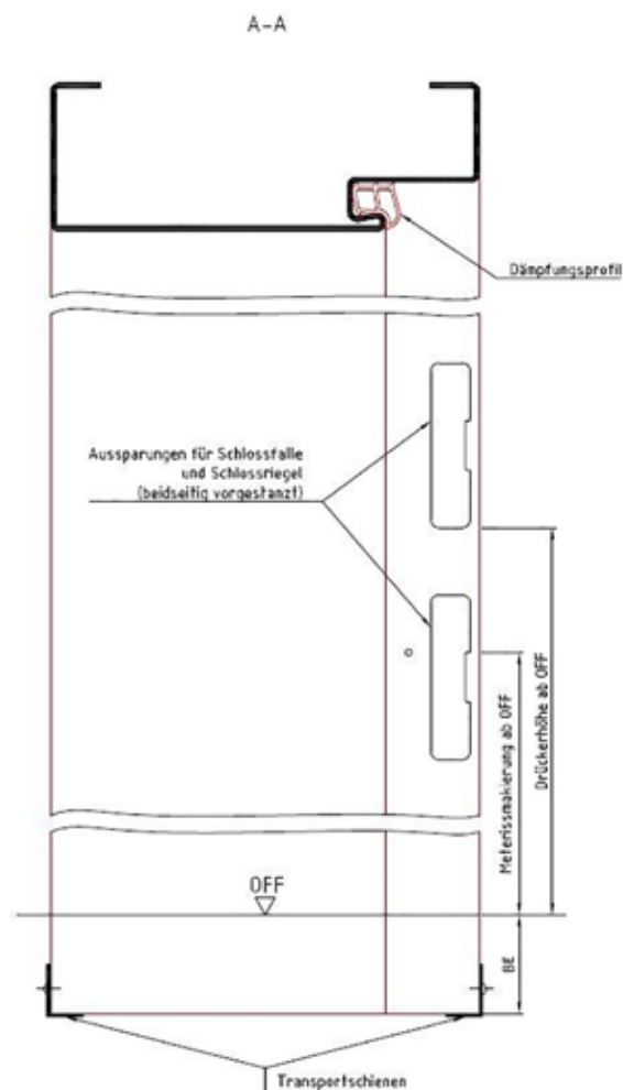
Bild 1 – wichtige Begriffe an einer Stahlzarge nach DIN 18111-1
