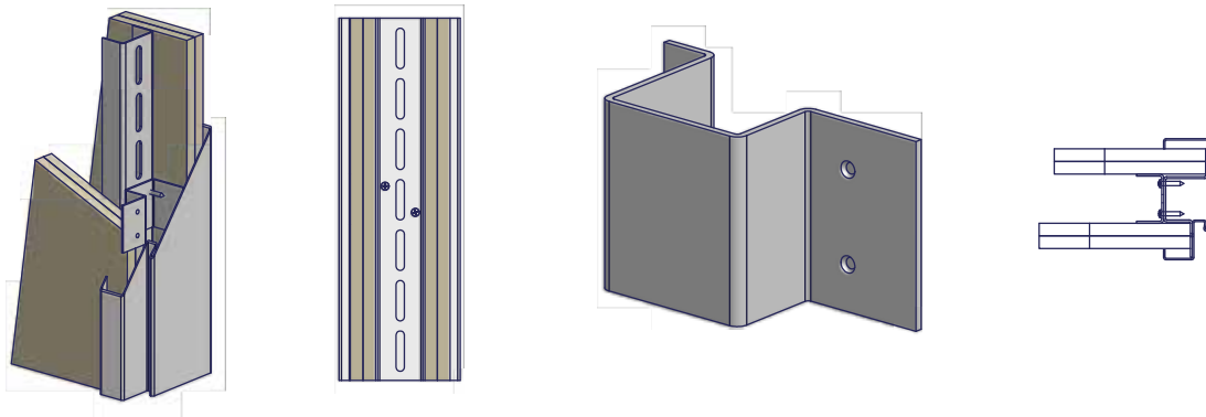
Bild 9 – Verwendung des Hutankers
