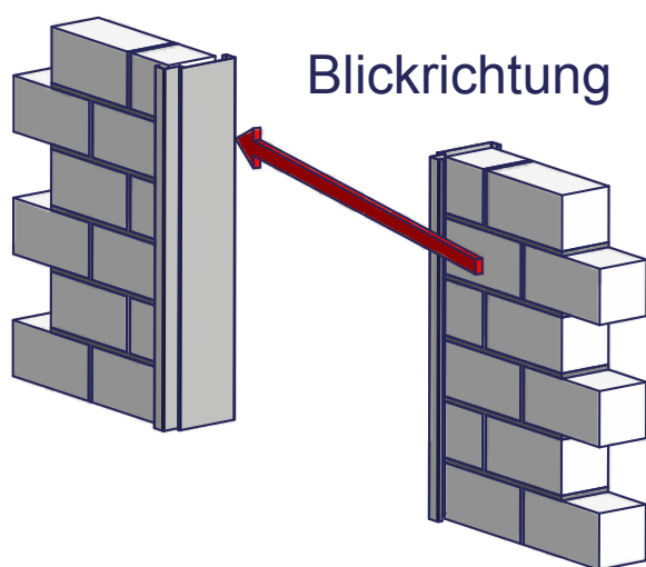
Bild 6a – Lotrechter Einbau von Stahlzargen
