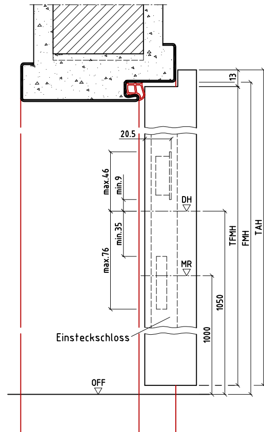
Vertikalschnitt
