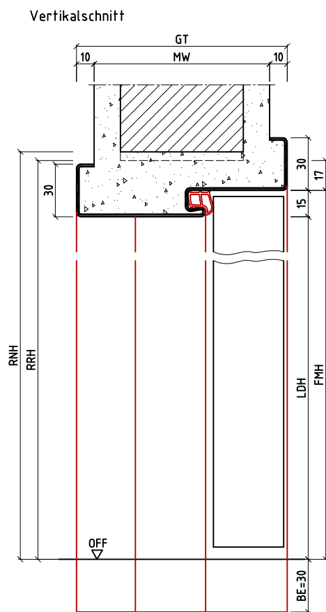
Darstellung Fall1
