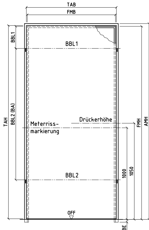
Ansicht
