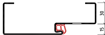
Schnitt B-B
