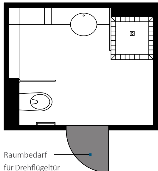
mit Drehflügeltür
