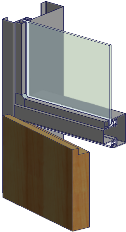
• Oberlichtzarge als H-Zarge (1-teilig) • für Mauerwerk oder Ständerwerk • andere Profilformen möglich
