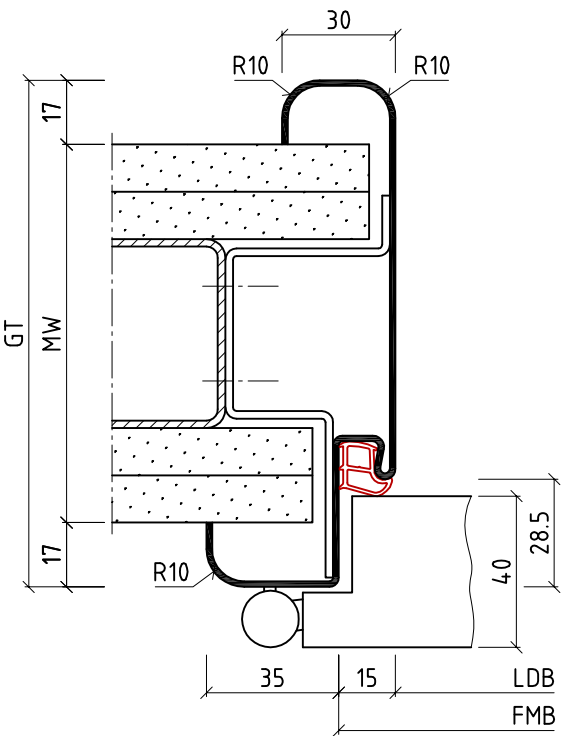
1rUud · Umfassungszarge mit Rundspiegel (1-teilig) · für Ständerwerk · Darstellung mit Bügelanker
