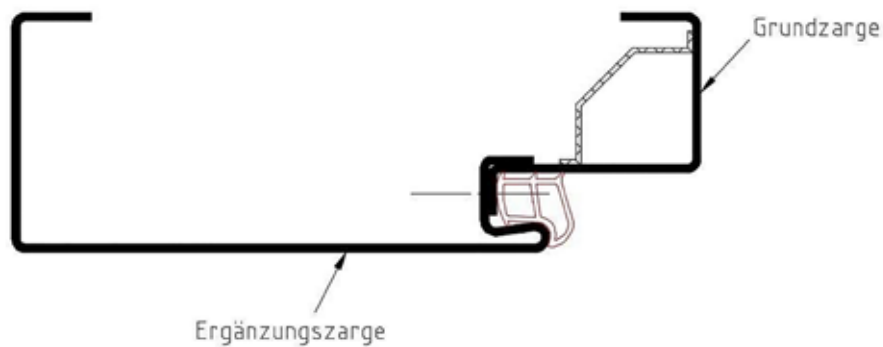
Bild 4 – Zargenprofil – 2-schalige Stahlzarge
