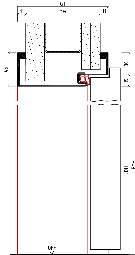
Vertikalschnitt
