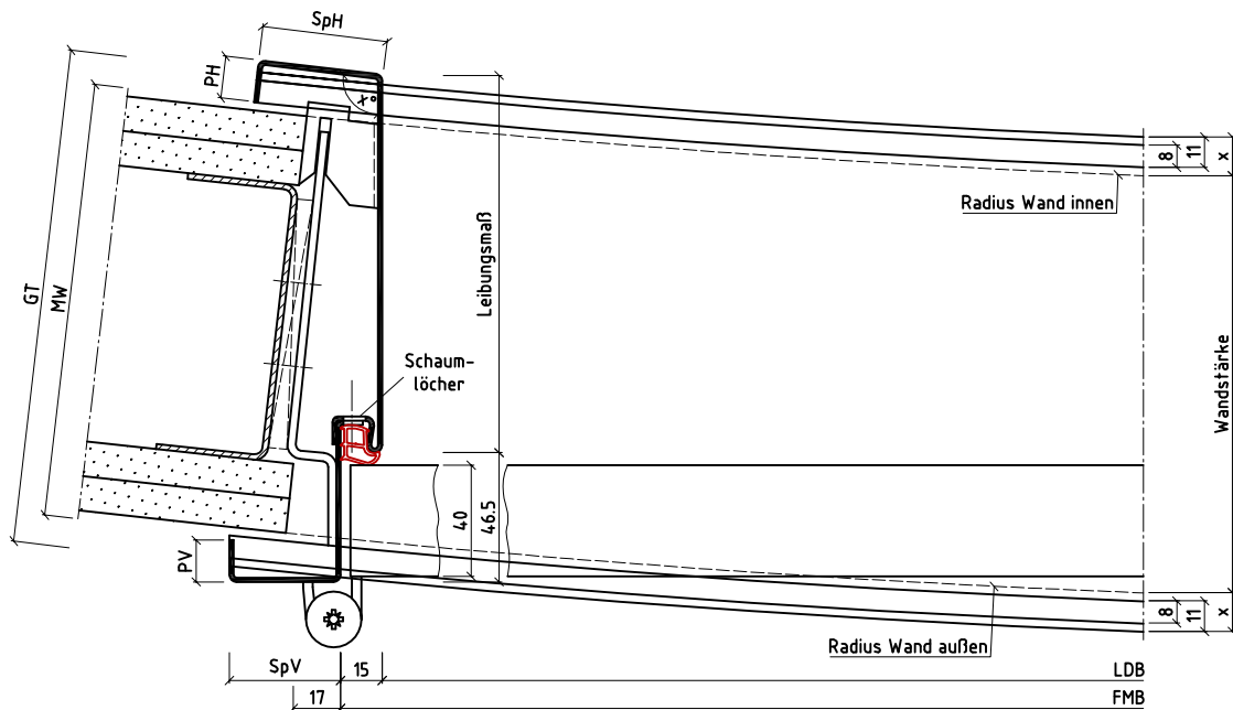
Horizontalschnitt
