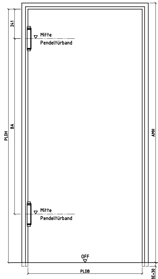
Ansicht
