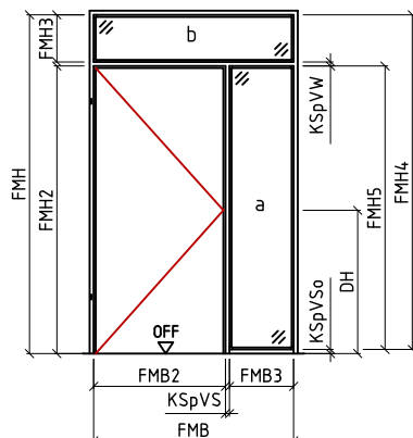
Oberlicht-/Seitenteilzarge
