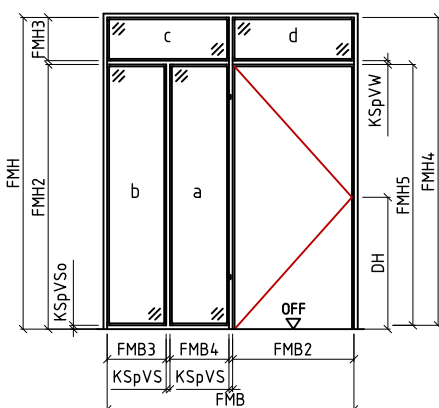
Oberlicht-/Seitenteilzarge
