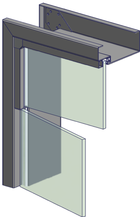
· Glasblendenzarge (1-teilig) · für Mauerwerk oder Ständerwerk · andere Profilformen möglich
