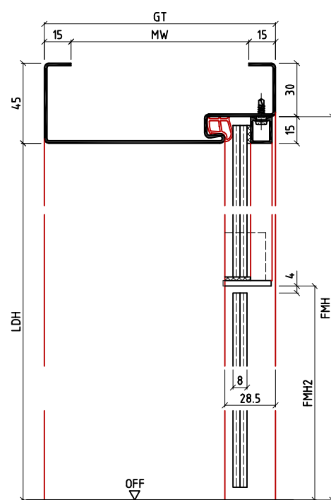
· Glasblendenzarge (1-teilig) · für Mauerwerk oder Ständerwerk · andere Abmessungen möglich
