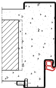
Potenzialausgleich Erdungsanschlussschraube M6 im BE-Bereich
