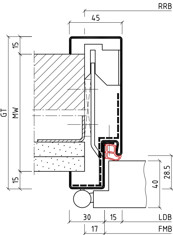
15ZBud · Umfassungszarge als Blockprofil mit Bleiteilauskleidung (2-schalig) · für nahezu alle Wandarten · Darstellung mit Flachstahlanker
