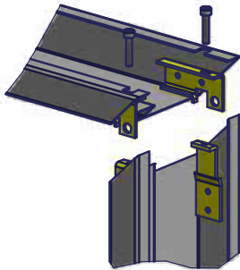
ECON3 Gehrungs- verbinding
