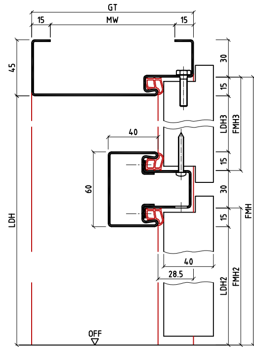
Bud/KEud · Holzblendenzarge (1-teilig) · für Mauerwerk oder Ständerwerk · andere Abmessungen möglich
