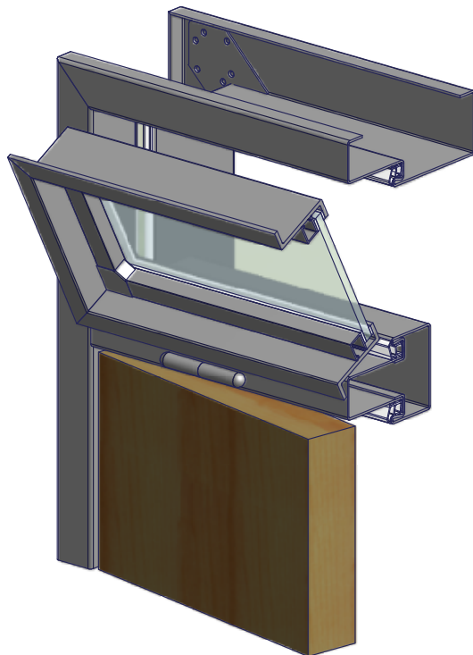
· Oberlichtzarge mit Kippflügel (1-teilig) · für Mauerwerk oder Ständerwerk · andere Profilformen möglich
