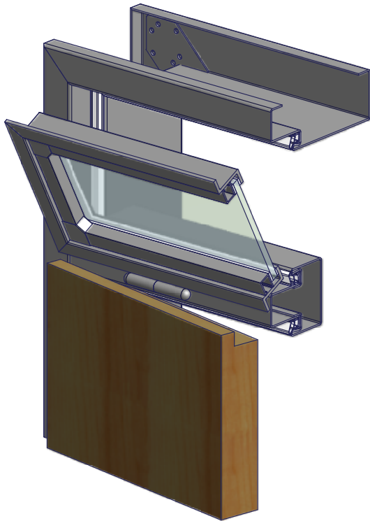
· Oberlichtzarge mit Kippflügel (1-teilig) · für Mauerwerk oder Ständerwerk · andere Profilformen möglich
