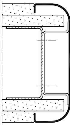
Wandabschlussprofil Typ 2
