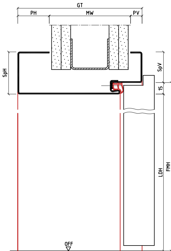
Vertikalschnitt
