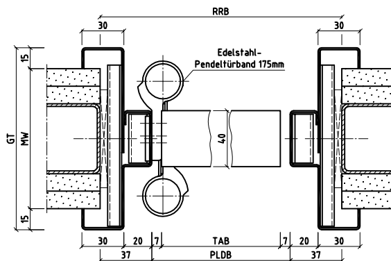
Horizontalschnitt
