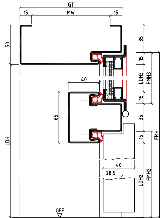
· Oberlichtzarge mit Kippflügel (1-teilig) · für Mauerwerk oder Ständerwerk · andere Abmessungen möglich
