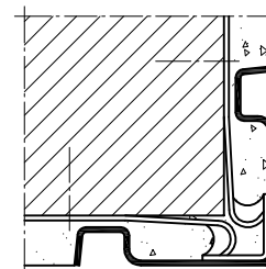
Eckschutzprofil Typ 3
