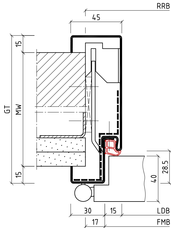
15ZBud · Umfassungszarge als Blockprofil mit Bleiteilauskleidung (2-schalig) · für nahezu alle Wandarten · Darstellung mit Flachstahllanker
