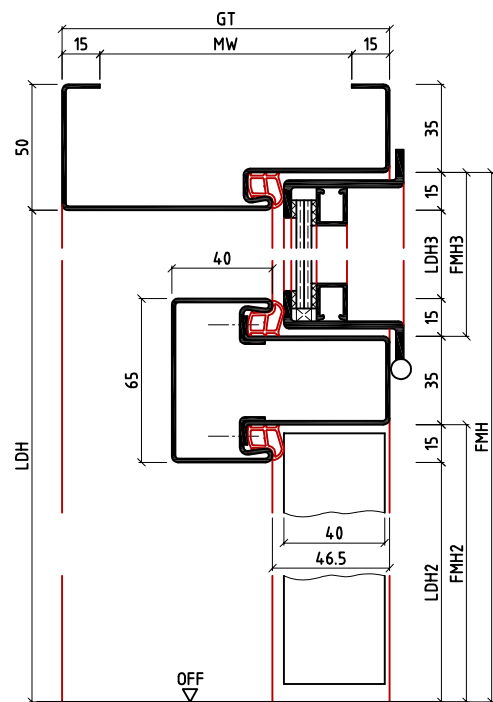
Bsd/KEsd · Oberlichtzarge mit Kippflügel (1-teilig) · für Mauerwerk oder Ständerwerk · andere Abmessungen möglich
