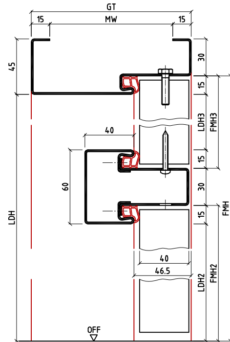
Bsd/KEsd · Holzblendenzarge (1-teilig) · für Mauerwerk oder Ständerwerk · andere Abmessungen möglich
