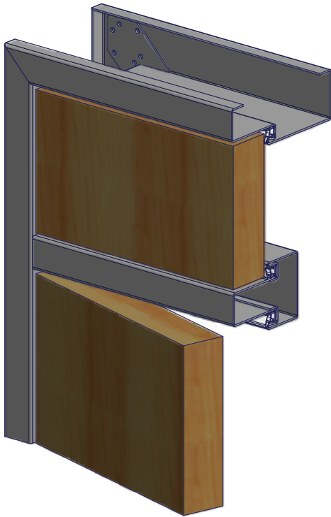
Bsd/KEsd · Holzblendenzarge (1-teilig) · für Mauerwerk oder Ständerwerk · andere Profilformen möglich
