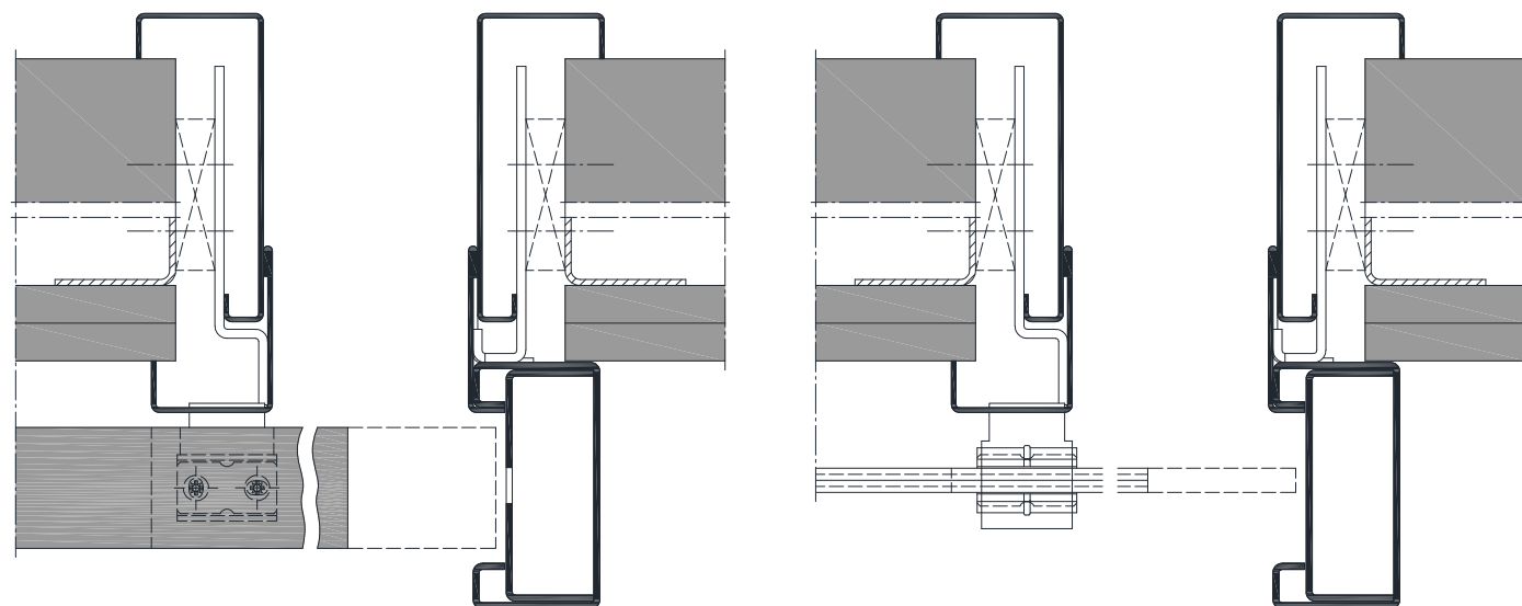
Holztürblatt
