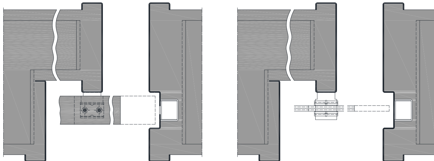
Holztürblatt
