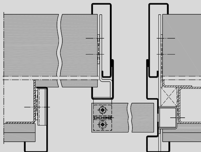
Variante mit Holztürblatt, Darstellung für Ständerwerk und Mauerwerk
