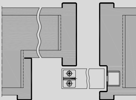
Variante mit Holztürblatt, Darstellung für Mauerwerk
