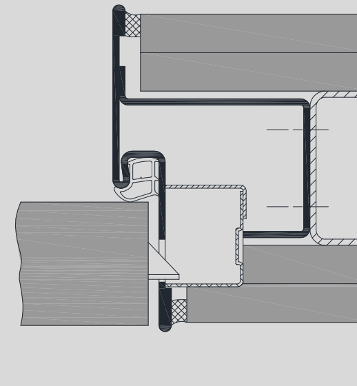
Oberlicht mit Rohrglasleisten
