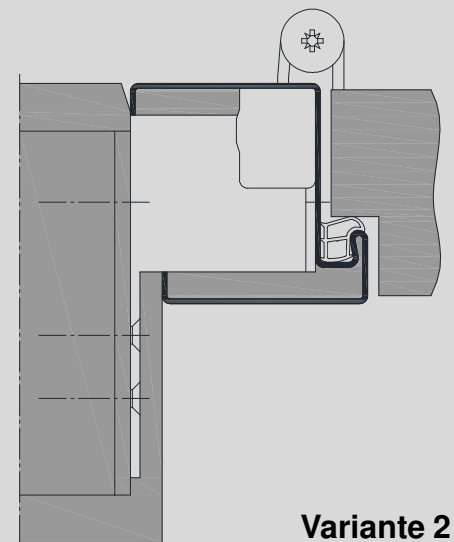
VX-Band, Variante 2 Oberlicht mit Rohrglasleisten
