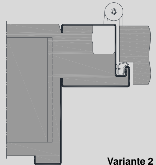
VX-Band, Variante 2 Oberlicht mit Rohrglasleisten
