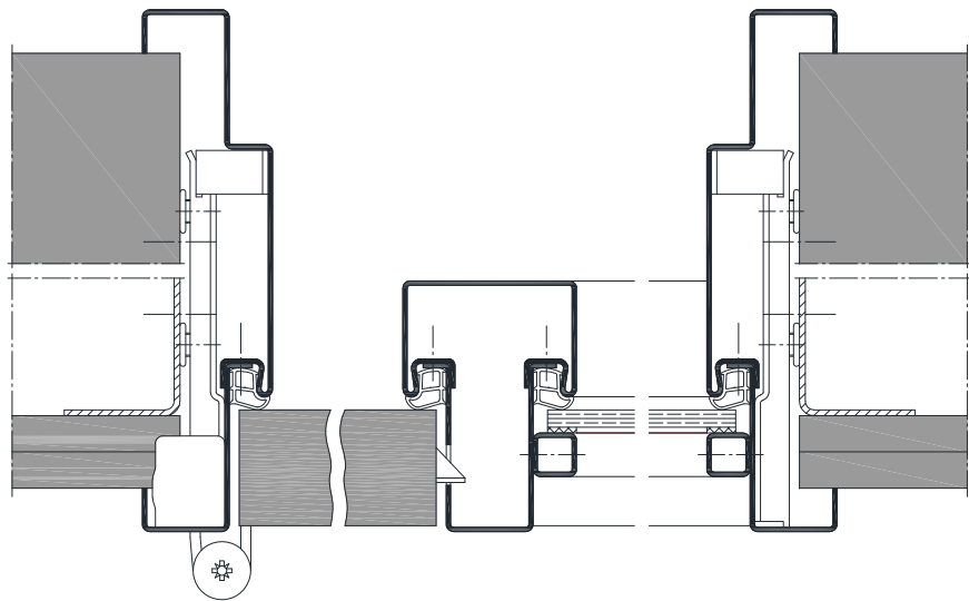
Seitenteil mit VX-Band
