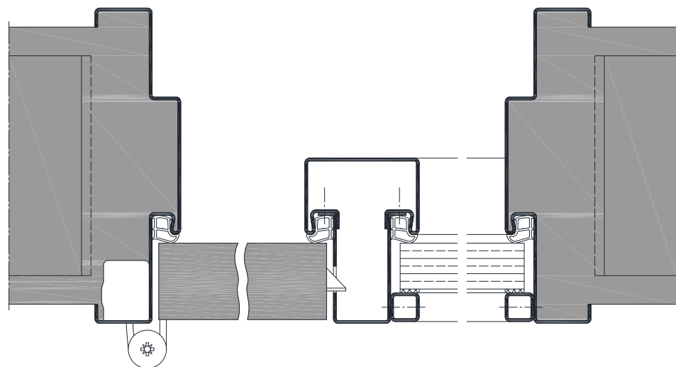
Seitenteil mit VX-Band
