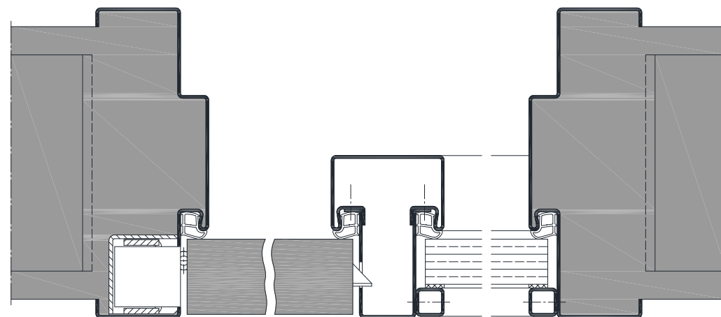
Oberlicht-/Seitenteil mit VX-Band
