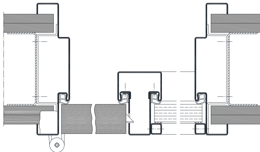
Seitenteil mit VX-Band
