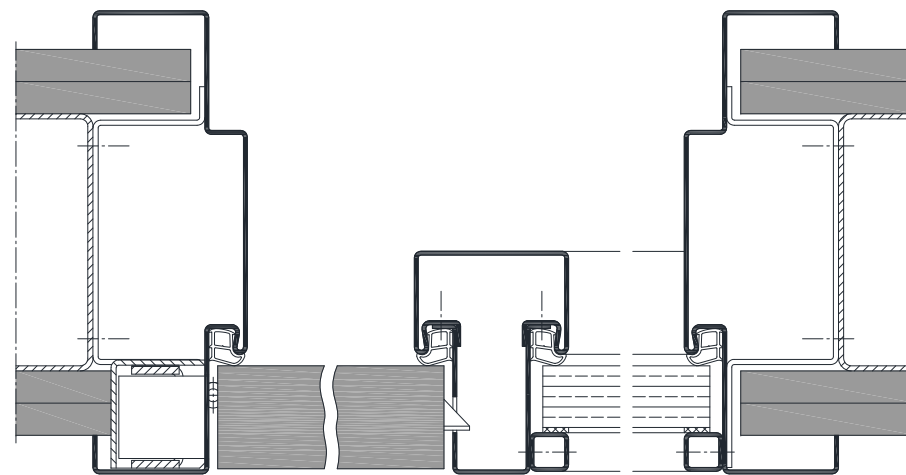
Oberlicht-/Seitenteil mit VX-Band
