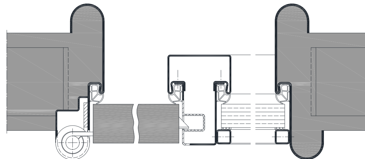
Oberlicht-/Seitenteil, inklusive Spezialbänder und Edelstahlschließblech
