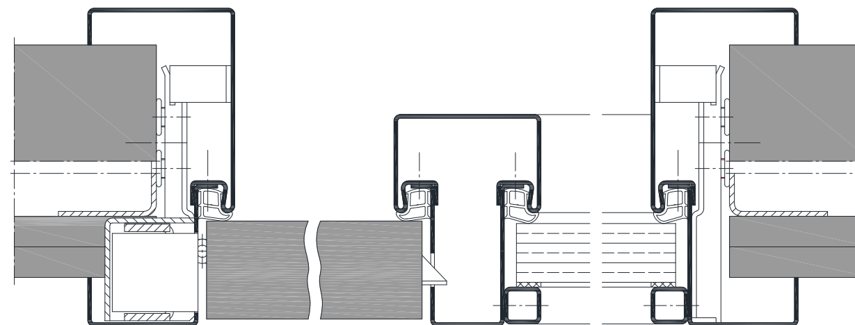
Oberlicht-/Seitenteil mit VX-Band
