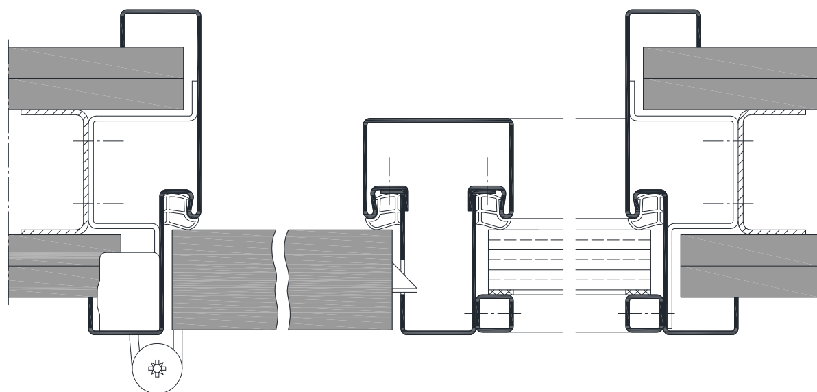
Seitenteil mit VX-Band
