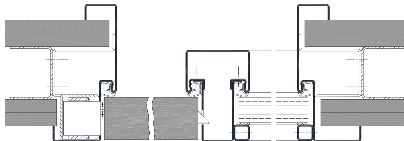
Oberlicht-/Seitenteil mit VX-Band
