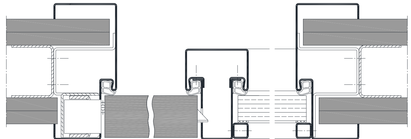
Oberlicht-/Seitenteil mit VX-Band
