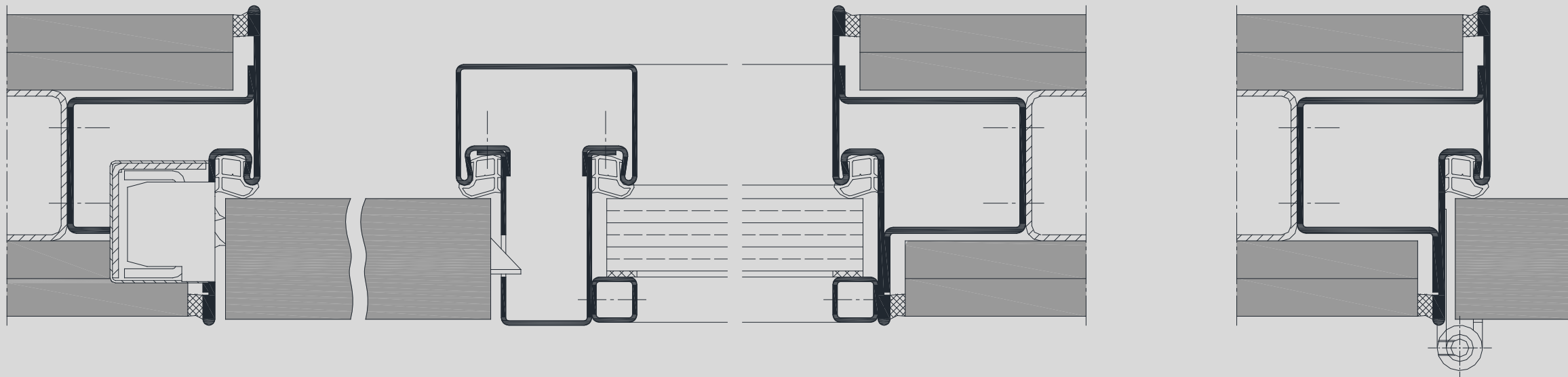
Varianten mit stumpf einschlagendem Türblatt, Darstellung für Ständerwerk
