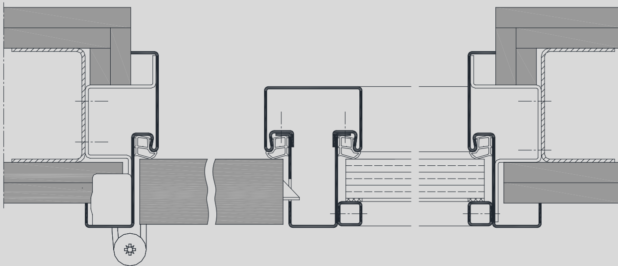
Varianten mit stumpf einschlagendem Türblatt, Darstellung für Ständerwerk
