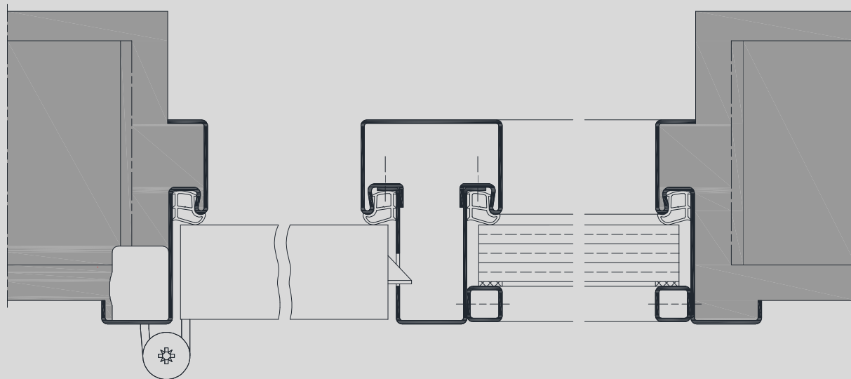
Varianten mit stumpf einschlagendem Türblatt, Darstellung für Mauerwerk
